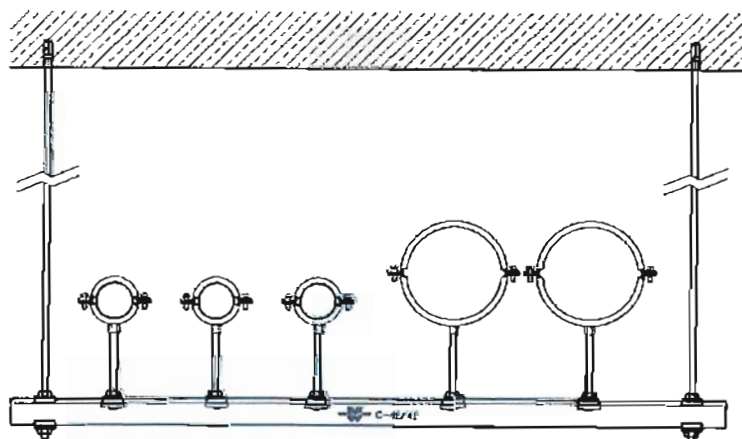
Abbildung 3-1: Schematische Darstellung abgehängt montierter Würth Varifix® C-Montageschiene, befestigt mit Gewindestangen und Muttern, Schrauben oder Dübeln der Dimension \geq M10 (Festigkeitsklasse \geq 4.6) mit brandschutztechnischem Nachweis in Verbindung mit Würth Halteklammern und Würth Hammerkopfschrauben, mit oberseitig montierten Installationen
