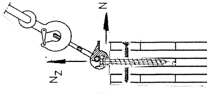
Bild 6: Quersugsicherung eines Brettsperrholzelements mit Vollgewindeschrauben
