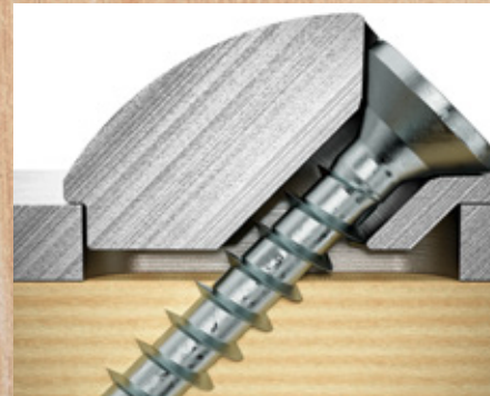
Winkelscheibe 45°
