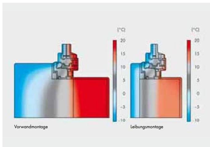
Abb. 1: Isothermenverlauf
