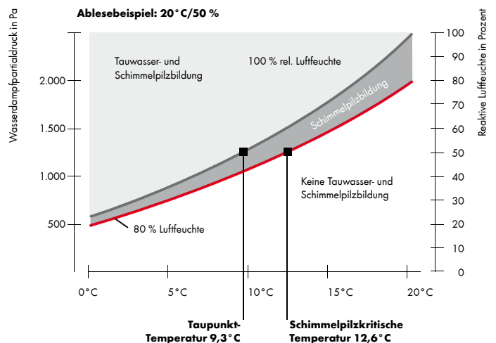
Abb. 2: Schimmelpilzkritische Temperatur
