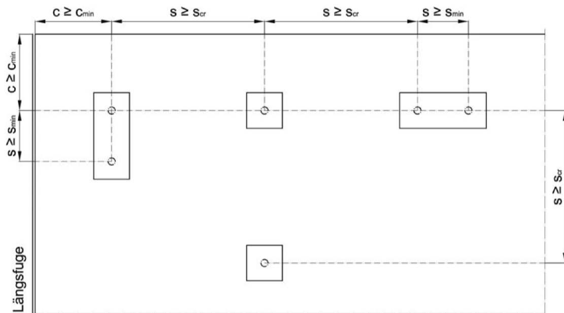
Abstände zwischen Dübelpaaren / Einzeldübeln
